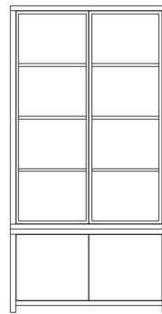
Cezar 2-Deurs/Vaks Enkele lijst 1230 B. 2162 H.
