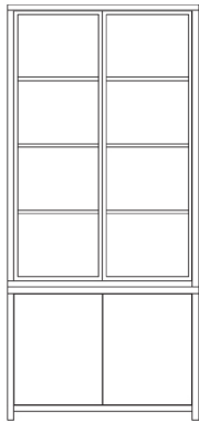
Cezar 2-Deurs/Vaks Enkele lijst 1230 B. 2362 H.
